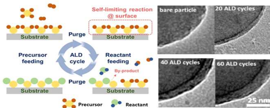
그림 14. ALD 공정의 Self-limiting 반응 메커니즘 및 cycle 기반 코팅층 성장 거동 (예시)
