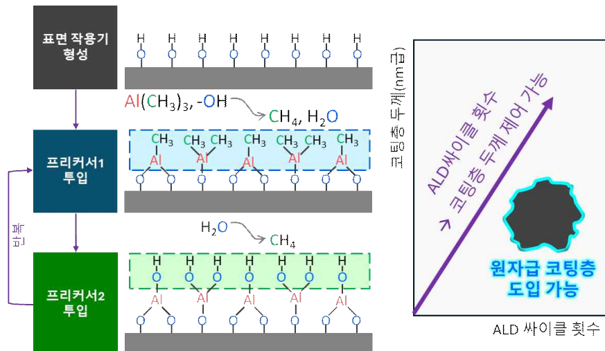
그림 12. 분말 ALD 나노 코팅의 기본 개념
