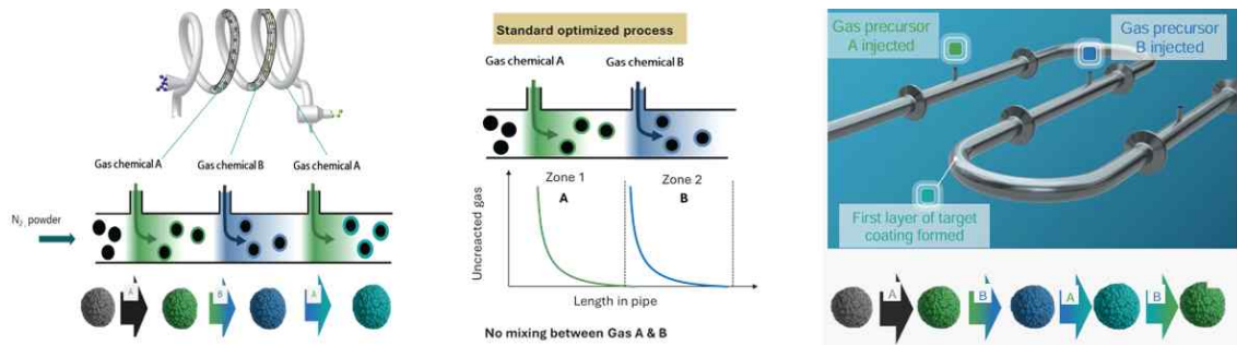
그림 15. 연속식 powder ALD 공정의 precursor distribution 및 coating 형성 개념
