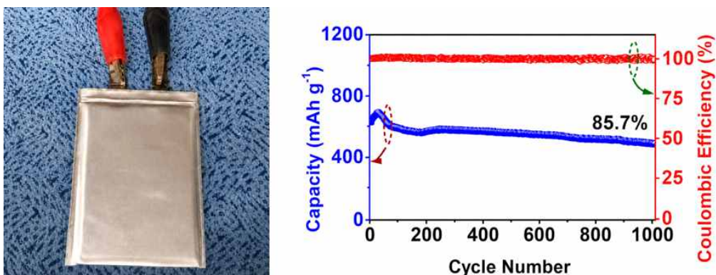
그림 25 Cycle 시험평가 결과 예시
